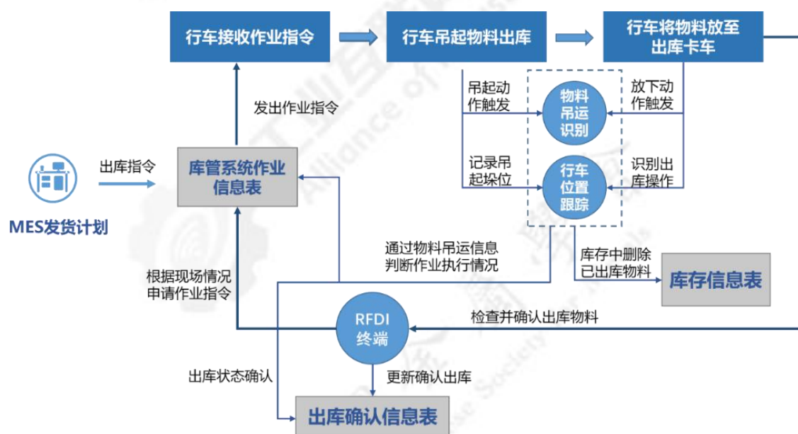
附图 2-2 无人行车和智能库管示意图
